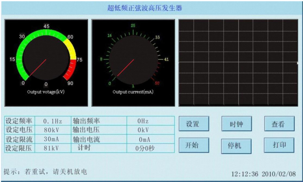
图 4 触摸屏示意图
